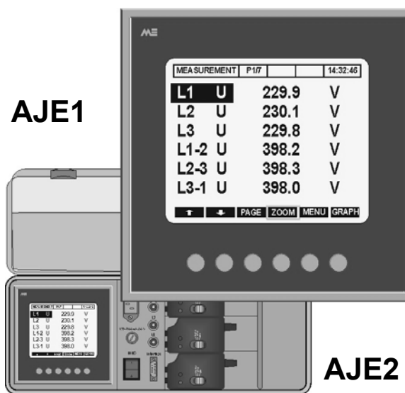
Rys. 4. Analizator jakości energii elektrycznej typu AJE1 i AJE2 (trójfazowe)
