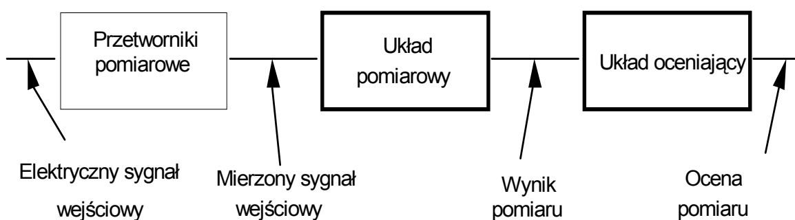
Rys. 1. Tor pomiarowy
