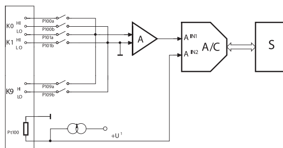
Rys. 2. Struktura układu do pomiaru temperatur miernika-rejestratora
