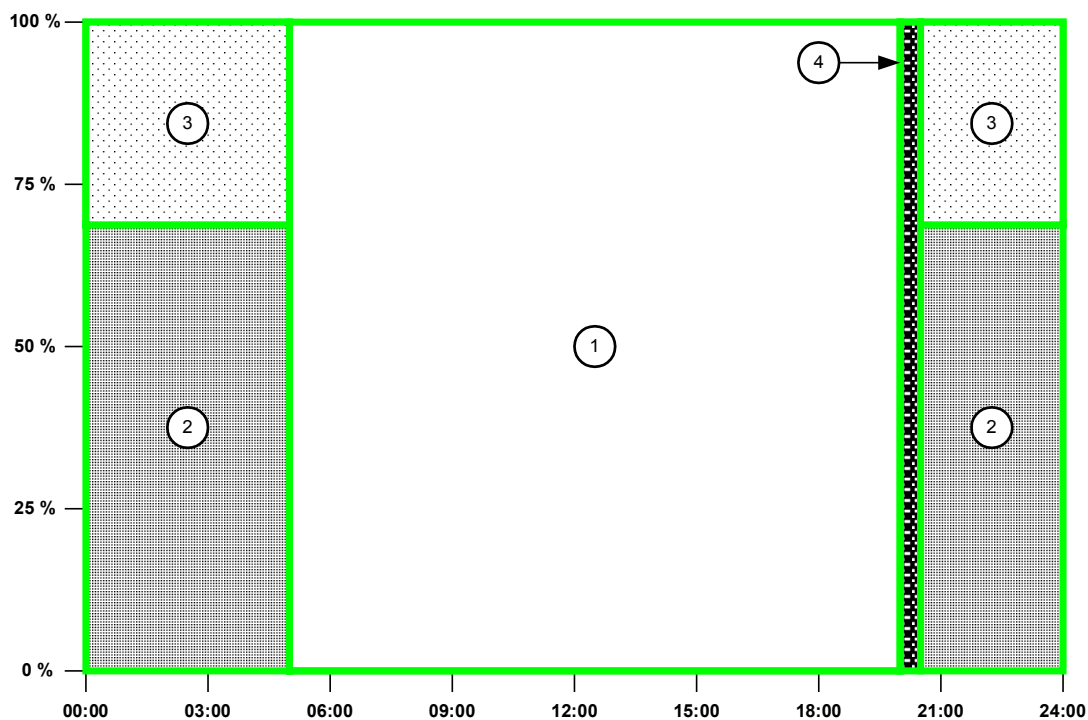
a) wykres dobowy redukcji przez ARZE1.T-16 poboru energii elektrycznej w okresie letnim
