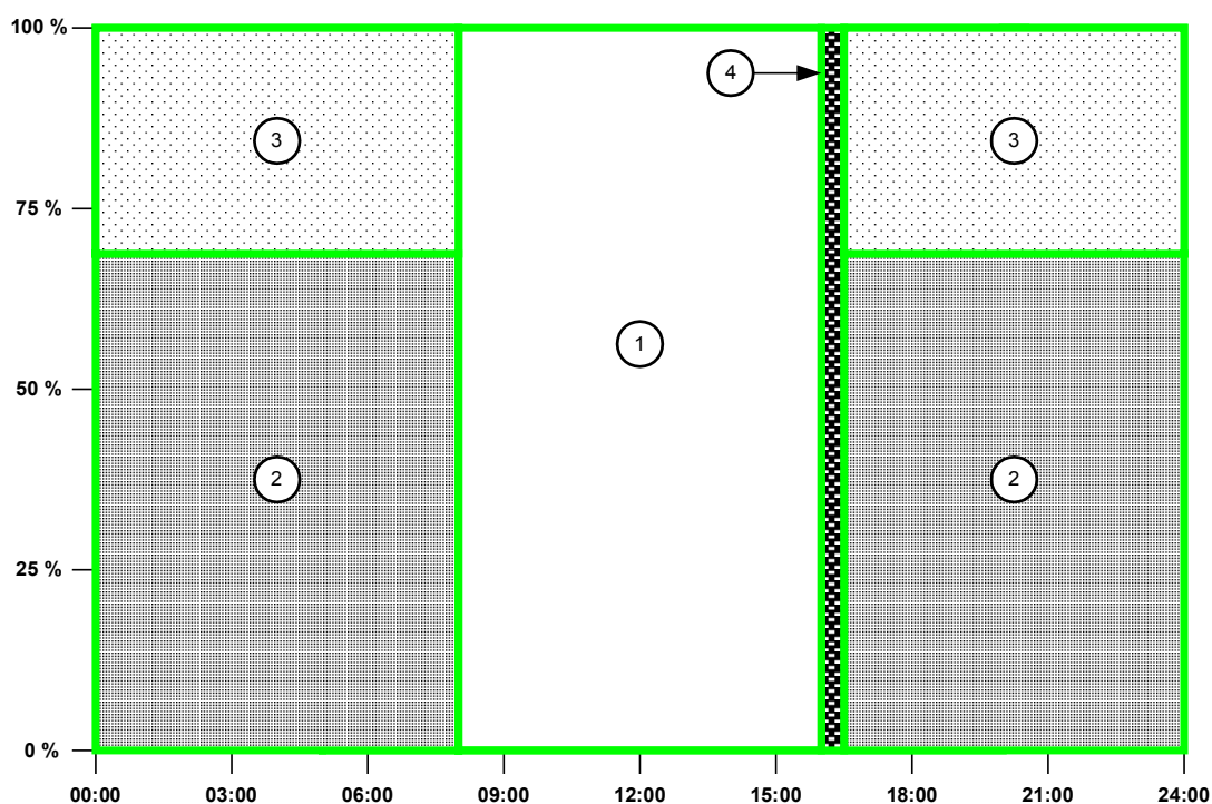
b) wykres dobowy redukcji przez ARZE1.T-16 poboru energii elektrycznej w okresie zimowym
