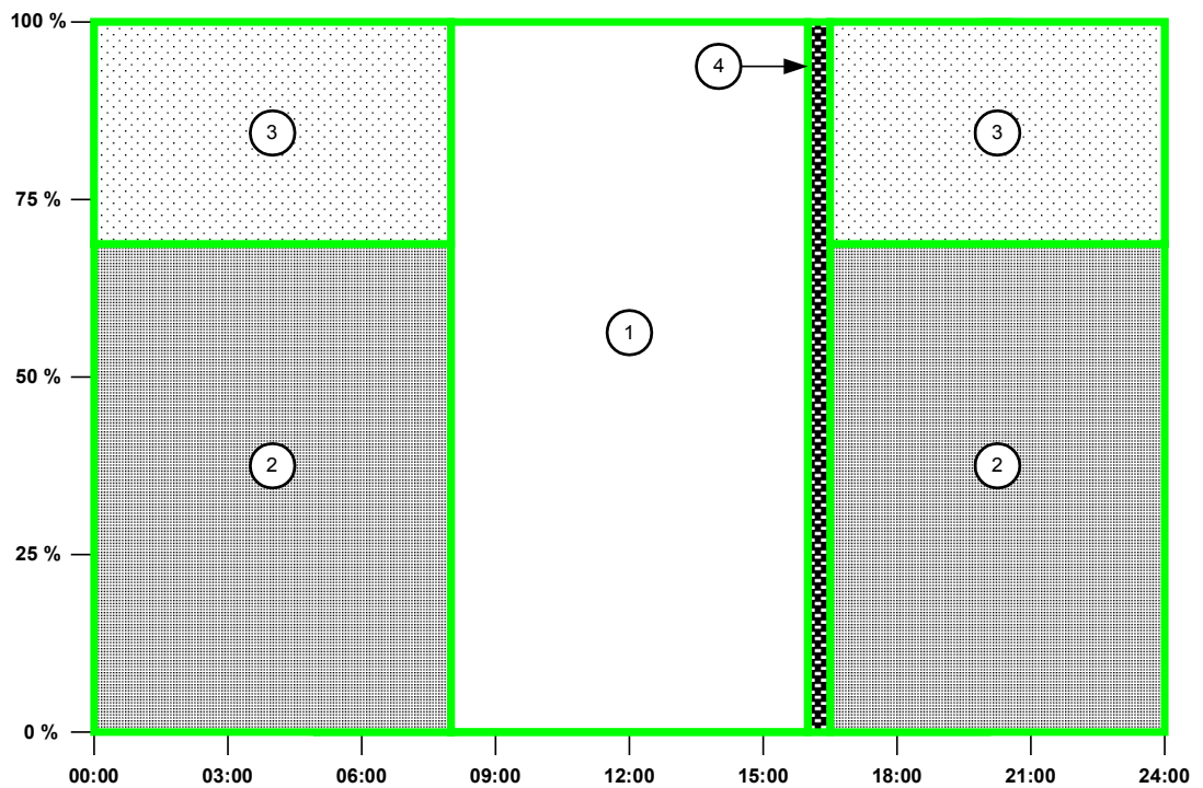
b) wykres dobowy redukcji przez ARZE1.T-10 poboru energii elektrycznej w okresie zimowym
